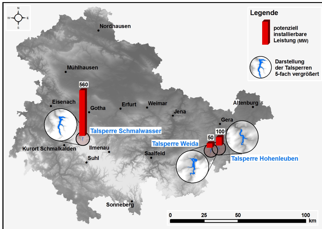
Abbildung 13: Leistungspotenzial an bestehenden Talsperren (Quelle: Hydroprojekt Ingenieurgesellschaft mbH, Datengrundlage: Thüringer Landesamt für Vermessung und Geoinformation)
