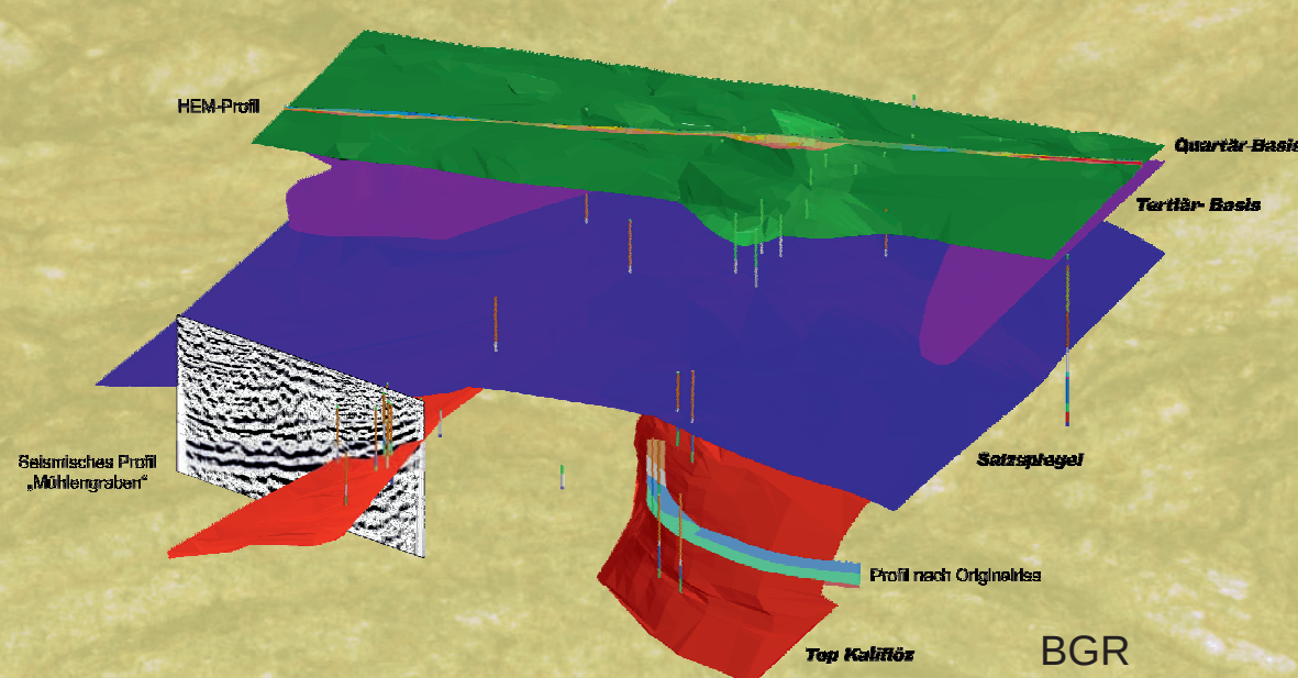
Geologisches 3D-Modell
